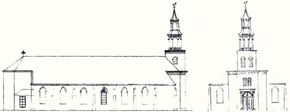
Schematische tekening van de St. Philippus & Jacobuskerk te Silvolde door Thomas H. von der Dunk op basis van het ontwerp van waterstaatsopzichter H. Bauer
